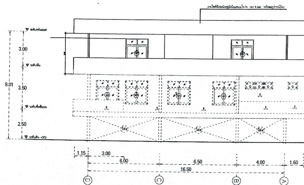
รูปด้าน 2 SCALE 1:100
