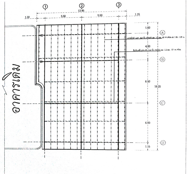
แปลนหลังคา SCALE 1:100
