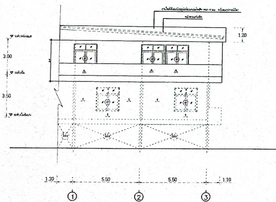
รูปด้าน 1 SCALE 1:100
