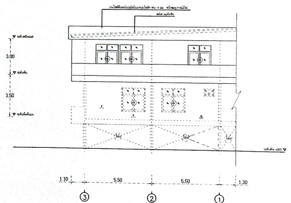
รูปด้าน 3 SCALE 1:100
