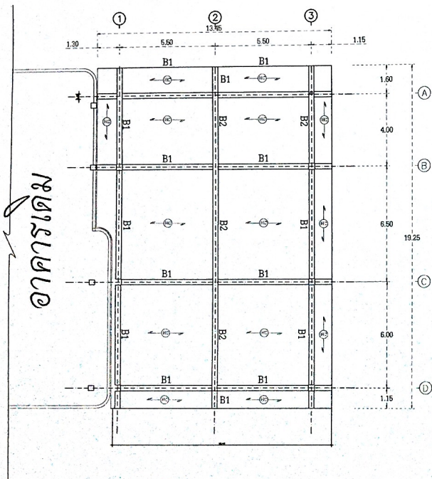
แปลนคาน้ำชั้น 3 SCALE 1:100
