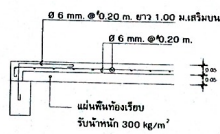
แบบขยายแผ่นพื้นช่วงริมคาน
