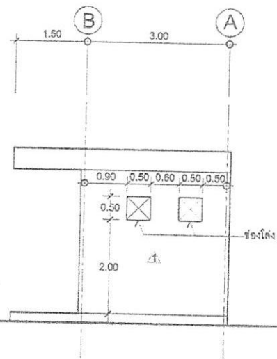
รูปด้านข้างขวา มาตราส่วน 1:75
