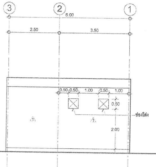
รูปด้านหลัง มาตราส่วน 1:75
