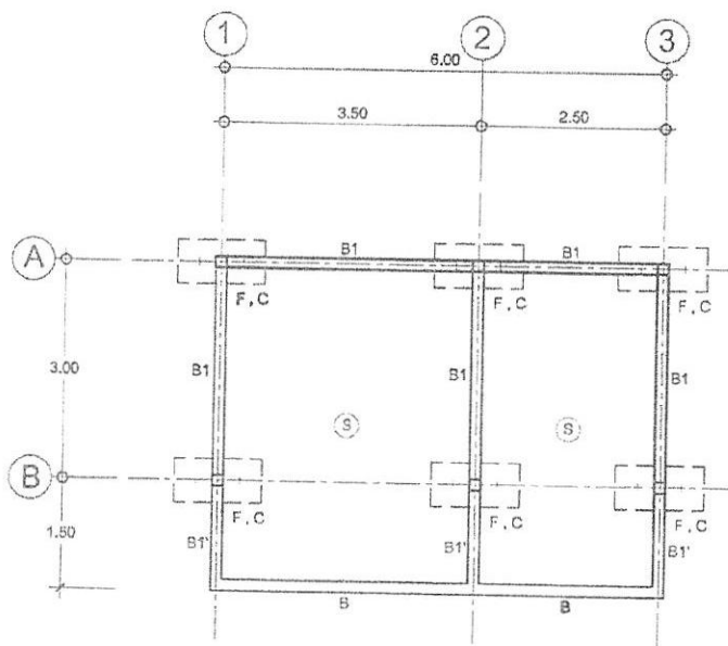
ผังฐานราก, เสา, คาน, พื้นชั้นล่าง (A) มาตราส่วน 1:75 S-01
