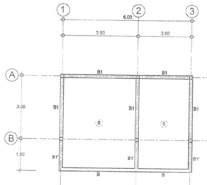
ผังคาน, พื้นชั้นหลังคา (B) มาตราส่วน 1:75 S-01
