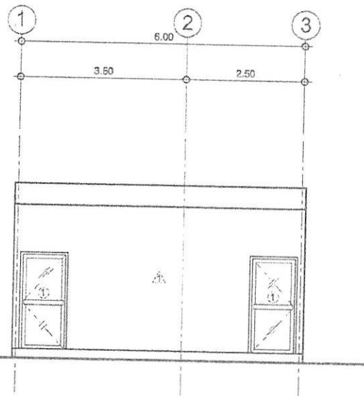
รูปด้านหน้า มาตราส่วน 1:75
